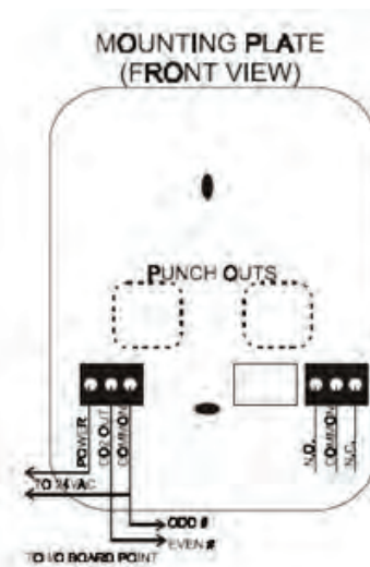
CO2 Sensor Wiring
