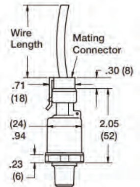
P/N 800-2XX0 Dimensions
