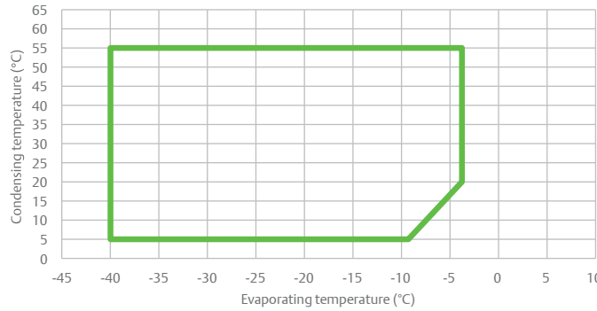
ZFI68-81KQE
