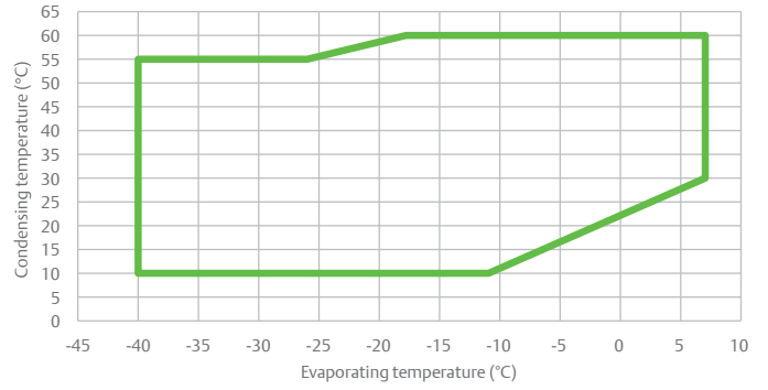
ZF25 - 41KQE
