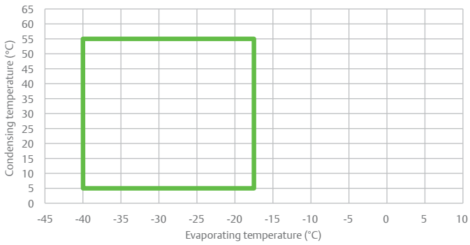
ZFI96-140KQE
